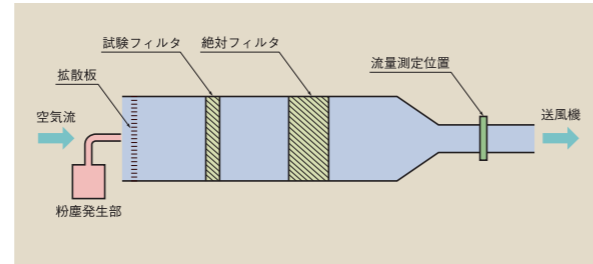
●質量法試験装置の例
